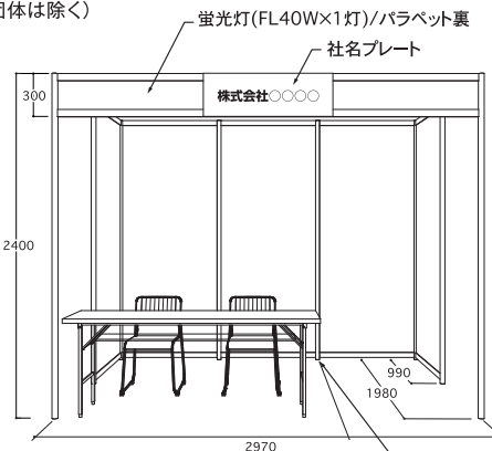
コンセント(2口)100V/300Wx1箇所
